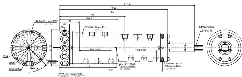
MK123S-S56 尺寸图 12进12出G3/8"牙
